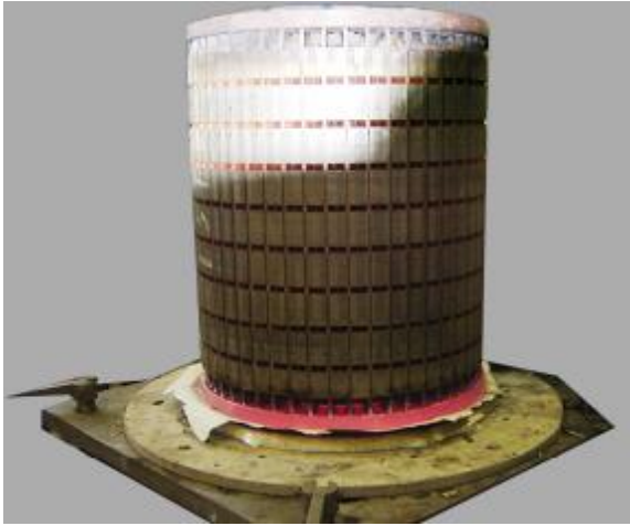
电机转子整体焊接
